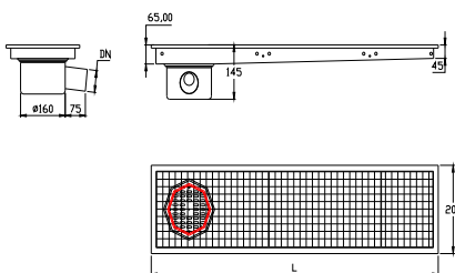
Bir Yöne Eğimli - Yandan Çıkışlı - Kenardan Sifonlu Çıkış Ölçüsü DN 50 - DN 70
