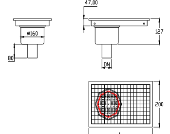
Eğimsiz - Alttan Çıkışlı - Kenardan Sifonlu Çıkış Ölçüsü DN 50 - DN 70
