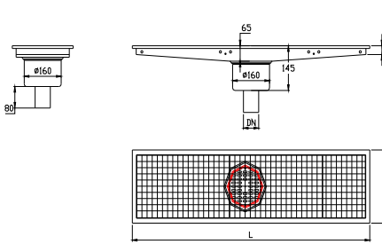
Ortaya Eğimli - Alttan Çıkışlı - Ortadan Sifonlu Çıkış Ölçüsü DN 50 - DN 70
