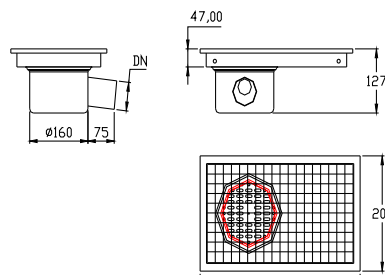
Eğimsiz - Yandan Çıkışlı - Kenardan Sifonlu Çıkış Ölçüsü DN 50 - DN 70
